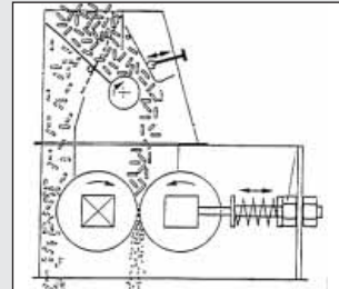
Roll Feeder 8 Serie
