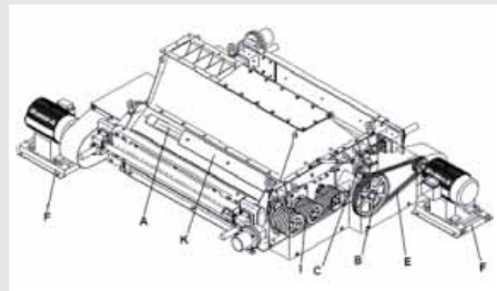
Roll Feeder 12 Serie
